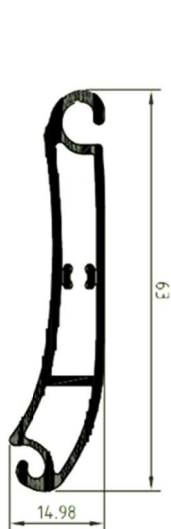
Lama autoblocante 60627
