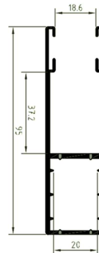
Guía autoblocante 95x27 50160
