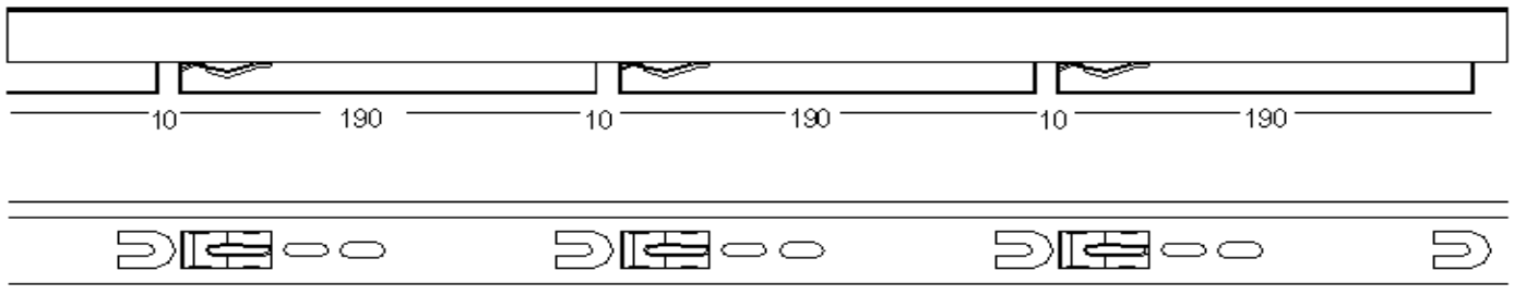
LAMA MONTADA CON SOPORTE PASO 200 PARA LCA
