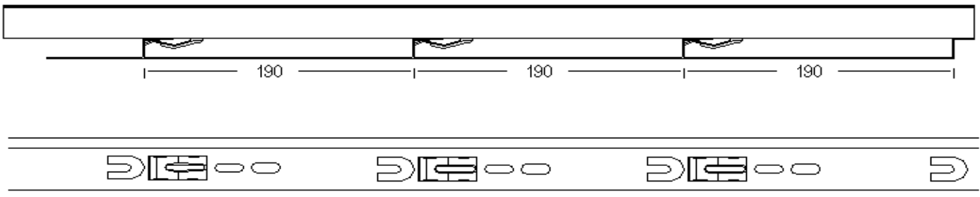
LAMA MONTADA CON SOPORTE PASO 190 PARA LCA
